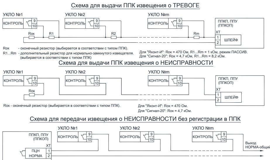
Рис. 4. Схема подключения УКЛО для контроля и трансляции сигнала неисправности линии оповещения.
