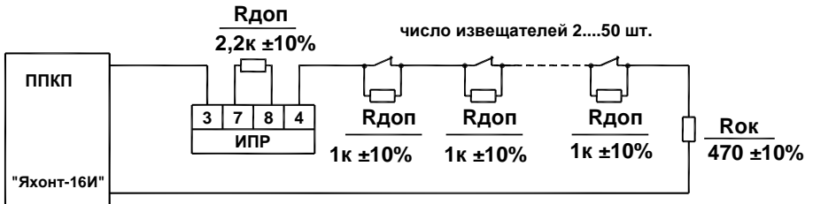
Тип ШС "ПАССИВ С ВНИМАНИЕМ"
