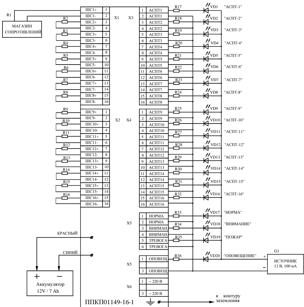
Схема внешних подключений прибора ППКП01149-16-1 при проведении общей проверки.
