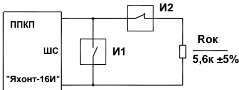
Только для ШС типа "ОХРАННЫЙ"
