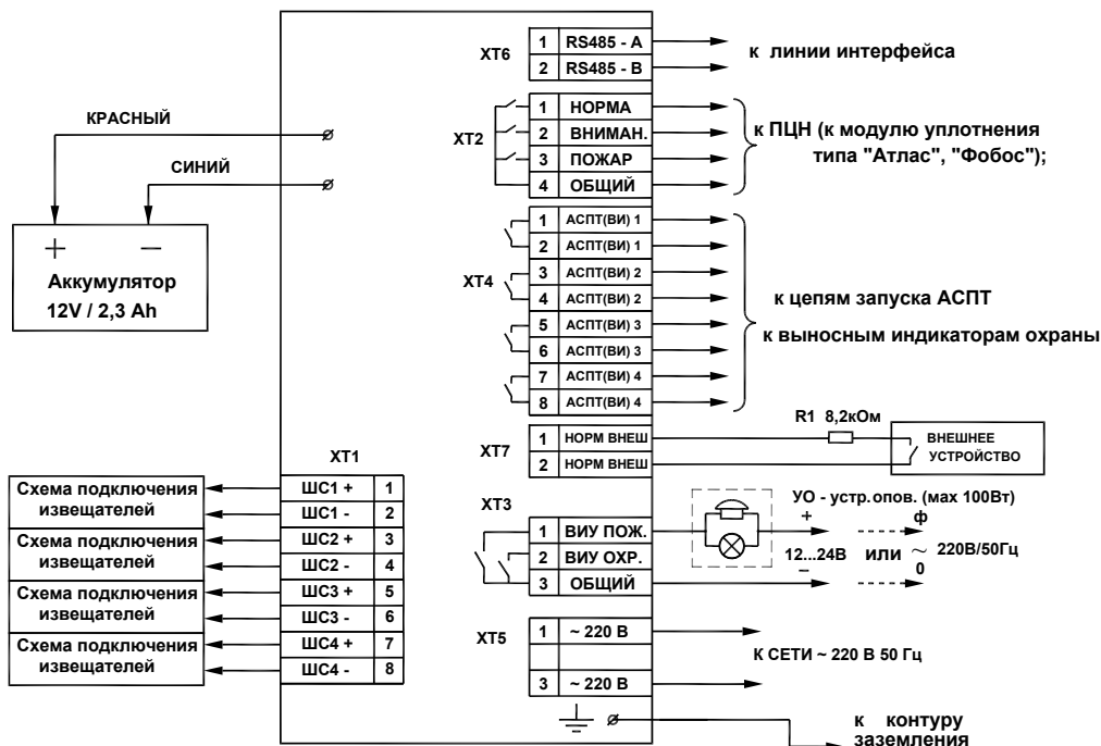
Схема внешних подключений прибора ПКОП01149-4-1 "Яхонт-4И"
