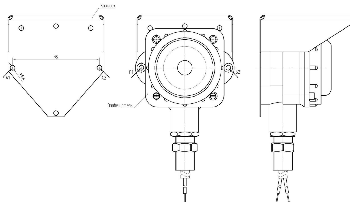
Рис. 4. Монтаж козырька с оповещателем «ЗОВ».
