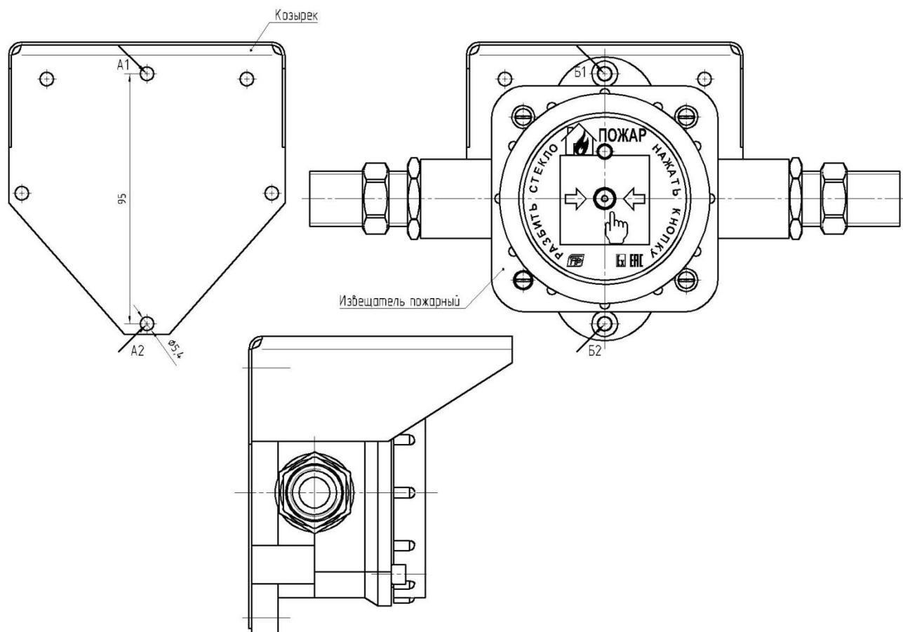
Рис. 3. Монтаж козырька с ИП «Гарант» двухвводный.
