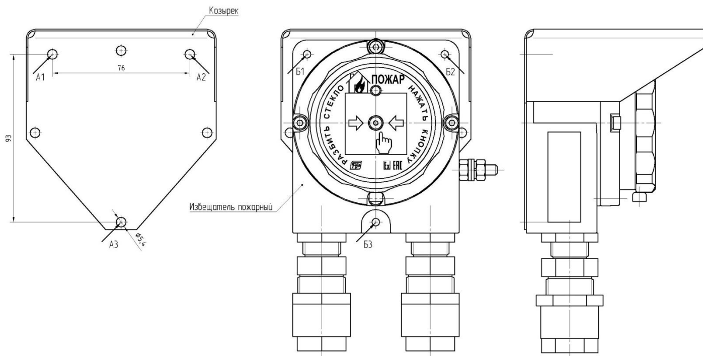
Рис. 2. Монтаж козырька с ИП «Гарант» однопроводный.
