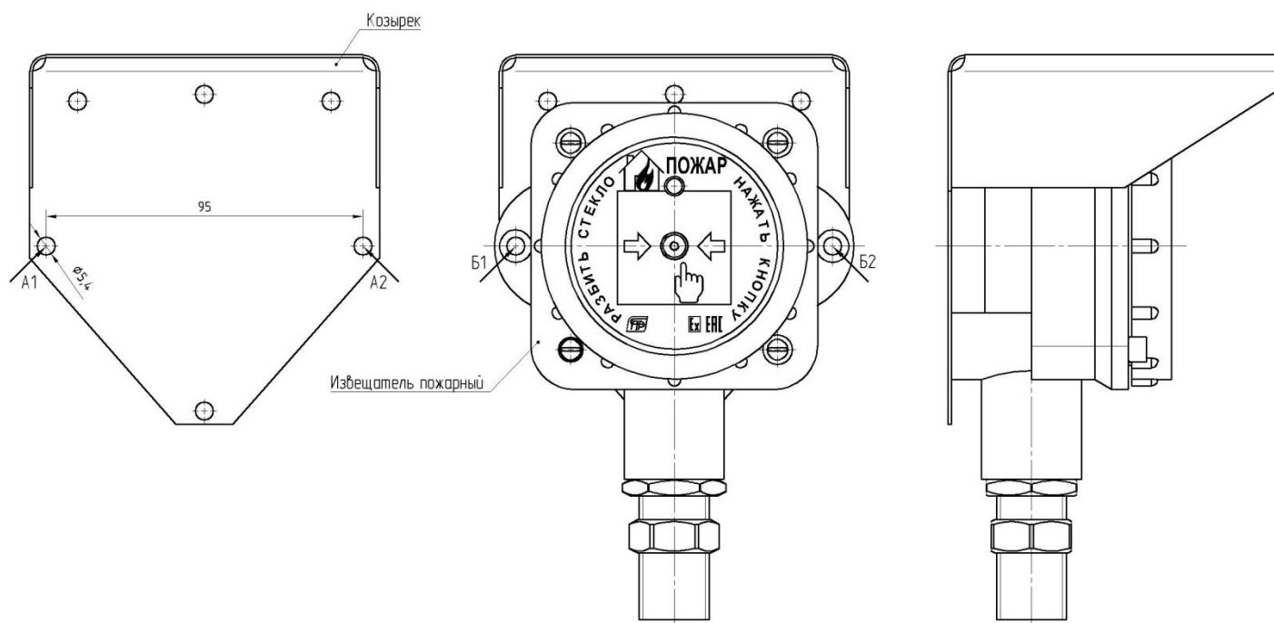
Рис. 2. Монтаж козырька с ИП «Гарант» однопроводный.
