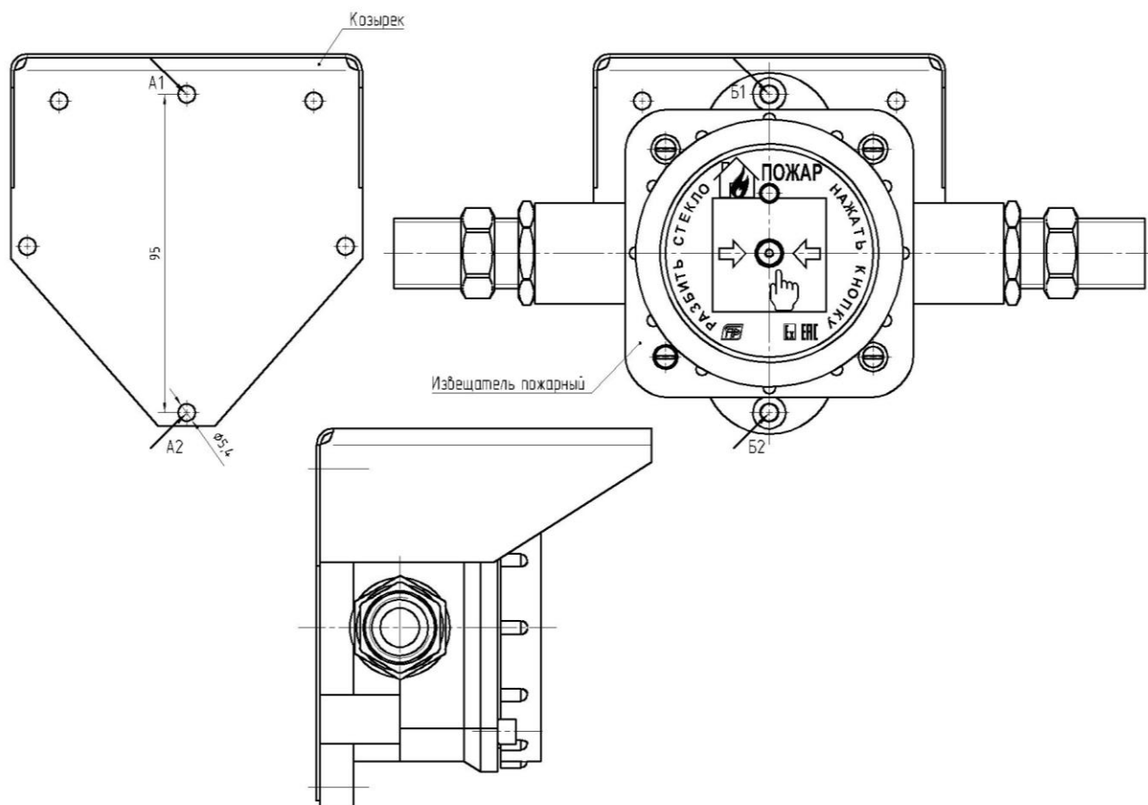
Рис 3. Монтаж козырька с ИП «Гарант» двухвводный.
